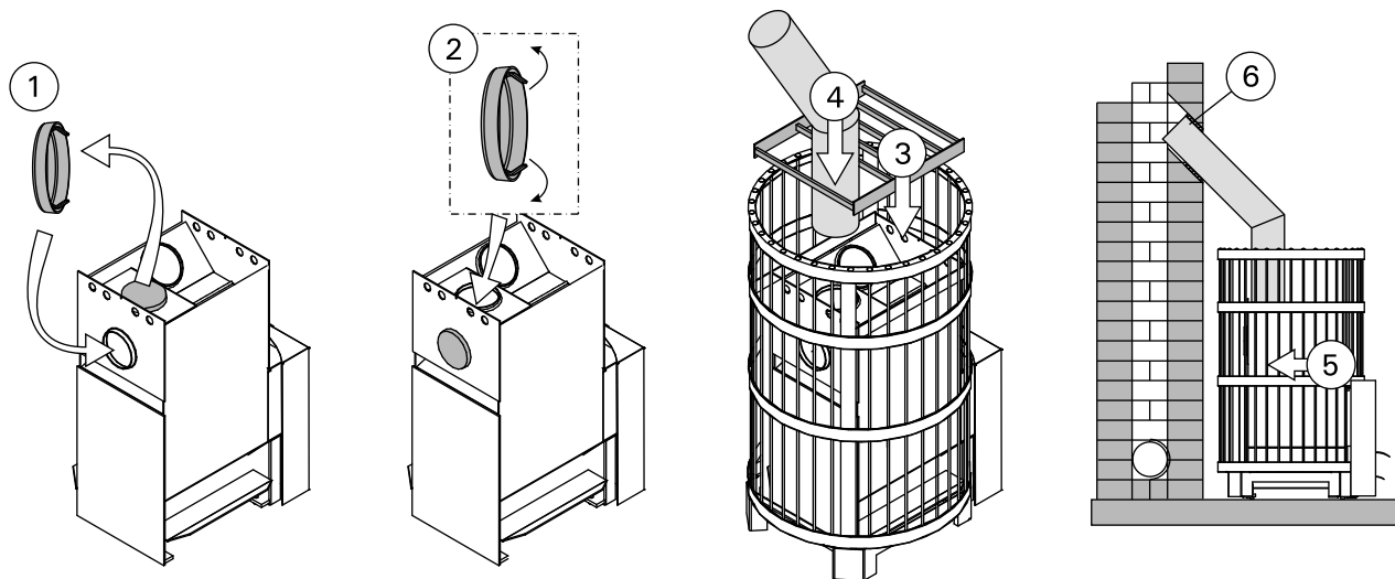
Рисунок 11. Присоединение каменки к каменному дымоходу через верхнее соединительное отверстие (все размеры приведены в миллиметрах)
