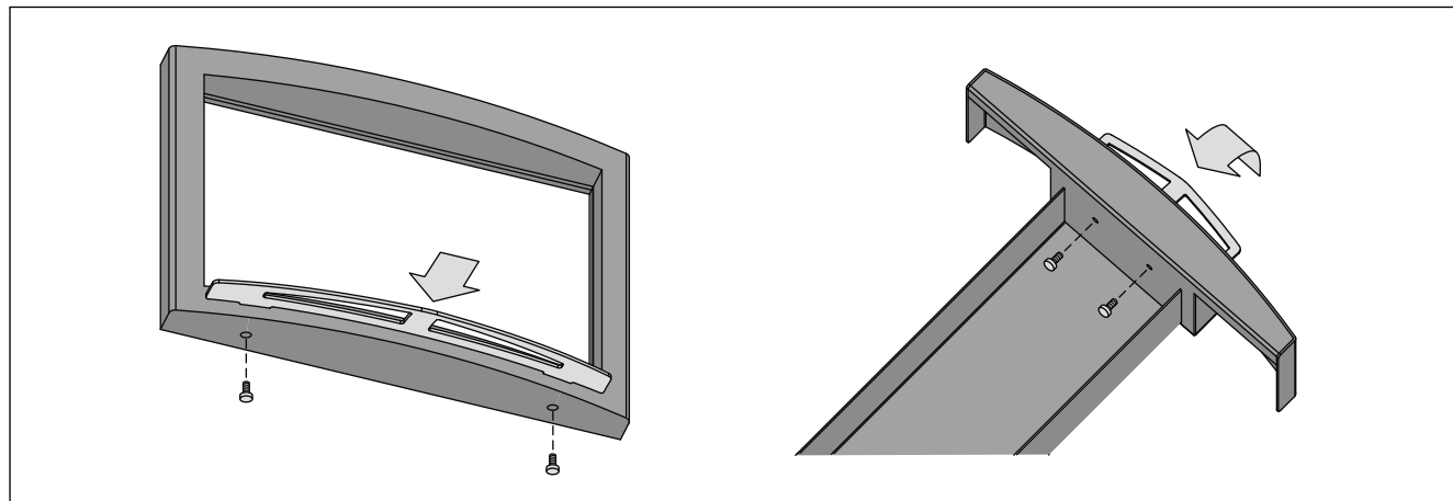
Рисунок 16. Установка ручяток (Legend 300)
